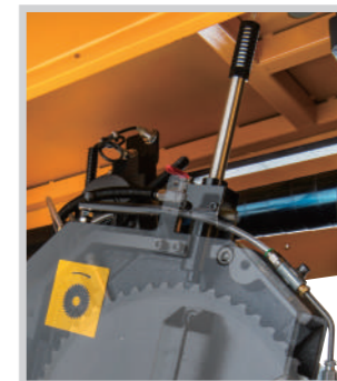
鋸片冷卻槍(選配)
