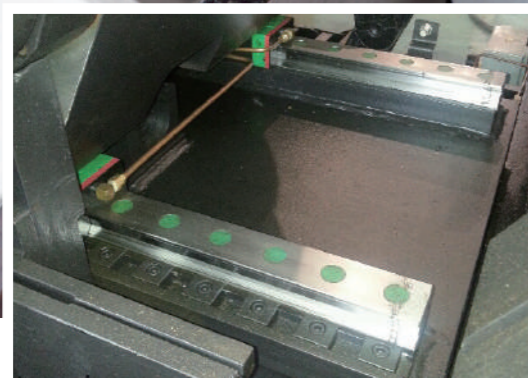
刀頭採用滾珠螺桿傳動，配合使用線性滑軌。
